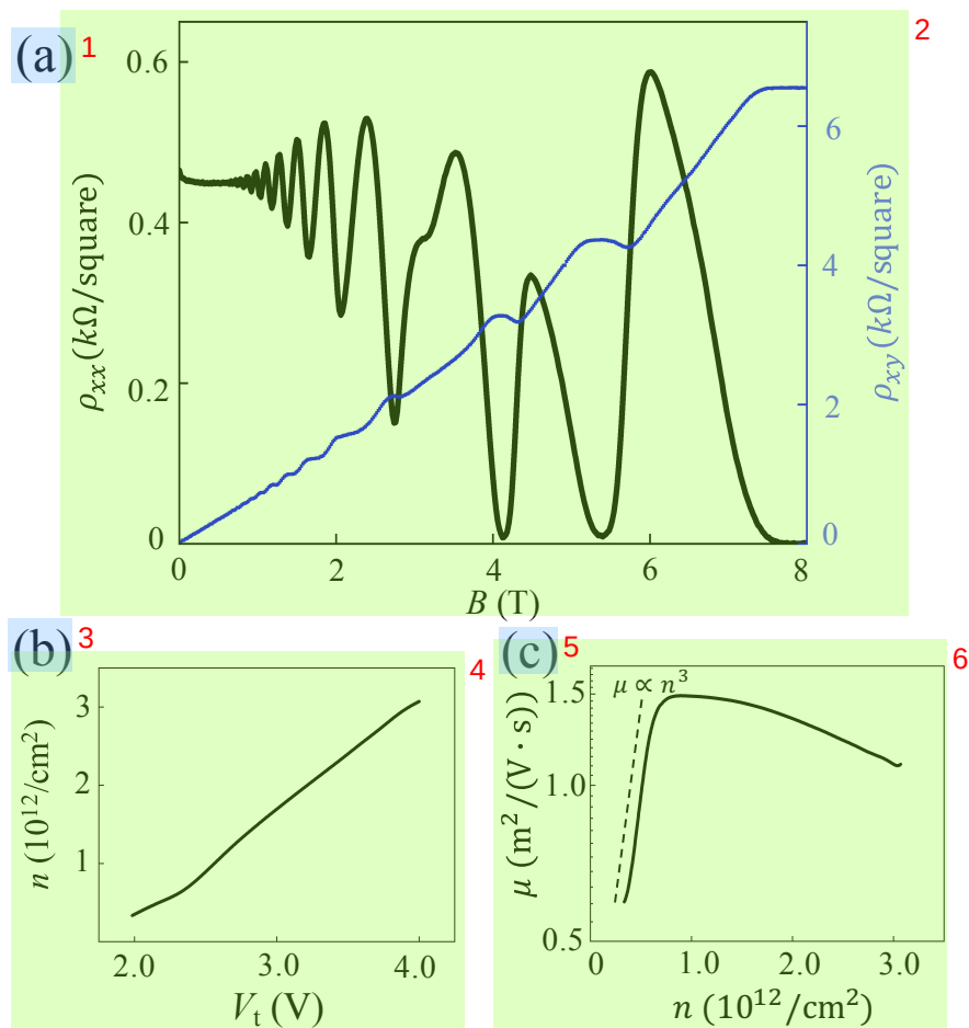
图 4.5 (a) 横向电阻率和纵向电阻率随磁场的变化。此时顶部栅压为 2.5 V，电子浓度为 9.06 \times 10^{11} \text{ cm}^{-2} 。(b) 电子浓度与顶部栅压之间关系。(c) 电子迁移率跟随浓度的变化关系。
