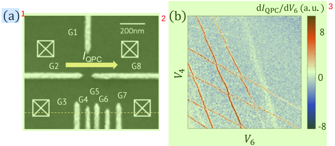
图 3.4 (a) 空穴型 GaAs 双量子点结构。(b) 使用电荷感应技术得到的电荷稳态图。测量的是 QPC 通道中电流 I_{QPC} 的微分电导 dI_{QPC}/dV_6 ，此时交流激励添加在 G6 上，白色带叉方块代表欧姆接触。
