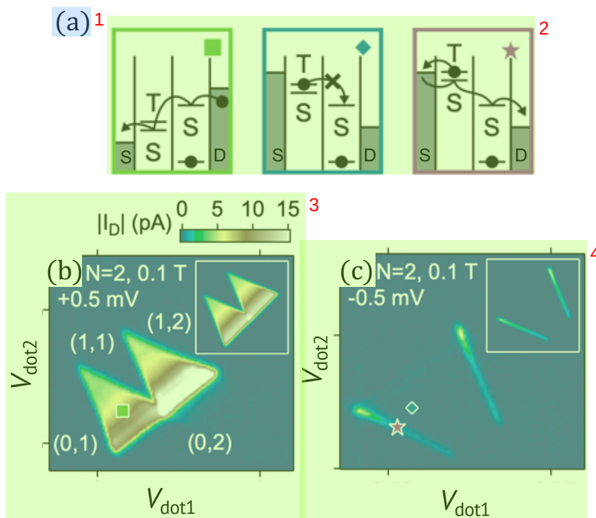
图 1.4 (a) 正负偏压下对应的能级图。三角形边缘及内部，在正偏压下电子从源极可以一直向左跃迁，形成向右的电流，在负偏压下只有跳跃到 S 态的电子才能完成跃迁循环，只要维持在 T 态，就无法完成向右的跃迁，形成向左的电流。(b) 正偏压下的电子数为 2 的偏压三角形。(c) 负偏压下的三角形。图片来自 [30]。
