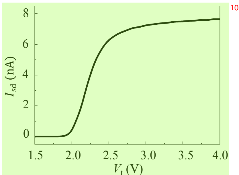
图 4.4 4.2 K 下两端法直接测量电流电压关系。外加的偏置电压为 20 \mu V。 11
