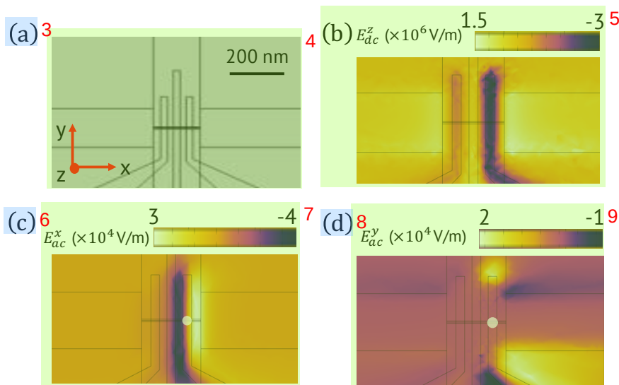
图 5.15 (a) 用于 COMSOL 计算的电极结构尺寸 (从 SEM 中获得)。(b) 直流电场在 z 方向的仿真结果。这里用到的参数有 V_L = 0.17 \text{ V} ， V_M = 0.085 \text{ V} ， V_R = 0.355 \text{ V} ， V_{sd} = 3 \text{ mV} 。(c) 和 (d) 不加直流电场，只考虑外加 0 dBm 功率的微波时，量子点处 (白色圆点) 受到的有效电场分别在 x 和 y 方向的分量大小。
