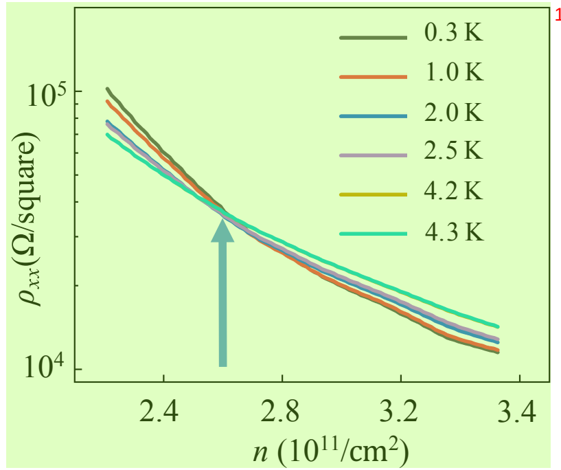
图 4.7 不同温度条件下，零磁场下横向电阻率随电子浓度的变化关系图。 2
