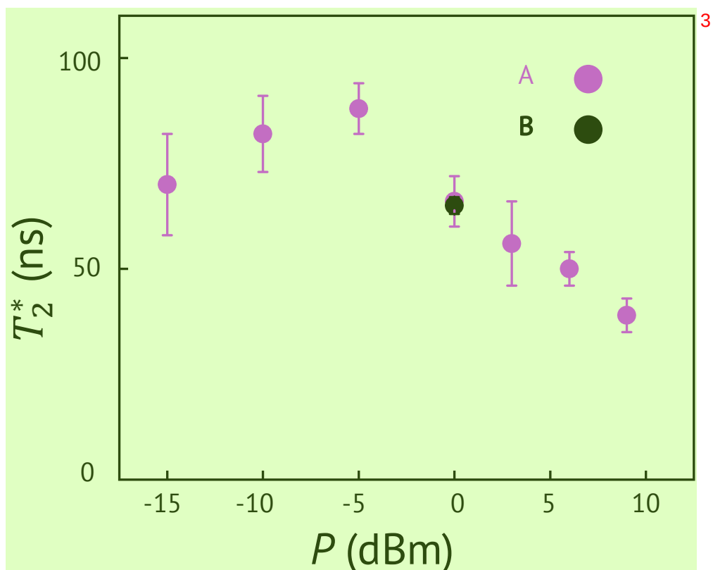
图 5.13 模式 B 在 0\text{ dBm} 时的退相干时间和模式 A 在不同功率下的退相干时间。 4
