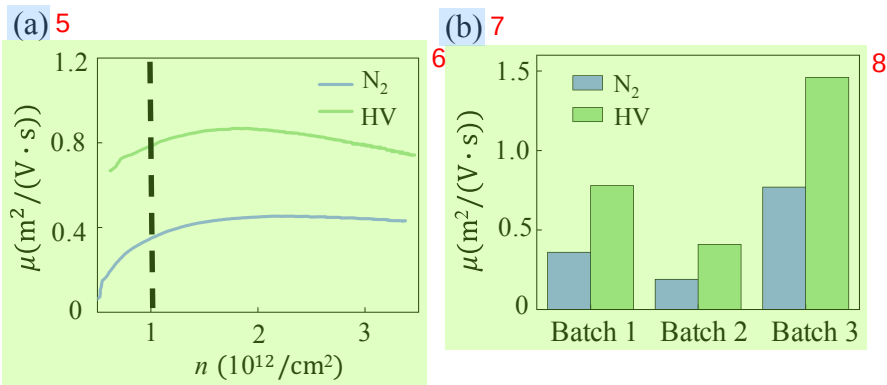
图 4.6 (a) 选取第一批次的样品，不同离子激活退火条件下的电子迁移率和电子浓度关系进行比较。(b) 三种批次，不同离子激活退火条件下获得的器件在电子浓度为 1 \times 10^{12} \text{ cm}^{-2} 时的电子迁移率对比。
