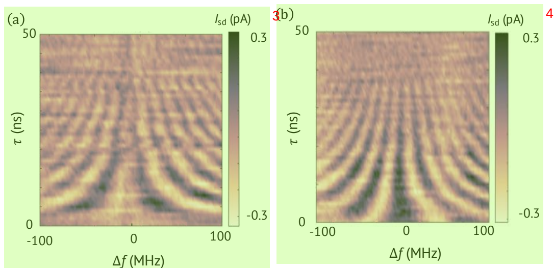
图 5.12 Ramsey 实验。(a) 两个 \pi/2 脉冲间的相位差为 \pi/2 时的情况。(b) 相位差为 0 的情况。此处的外加功率为 -10 dBm。 5
