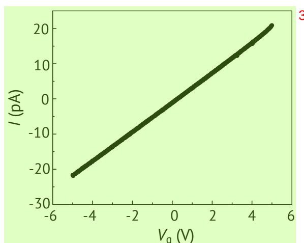
图 2.4 GaAs 基片上的漏电流测试。直流电压接顶部栅极，万用表接下层电极，栅极和下层之间由绝缘层隔绝，如果绝缘性质良好，将不会测得电流变化。
