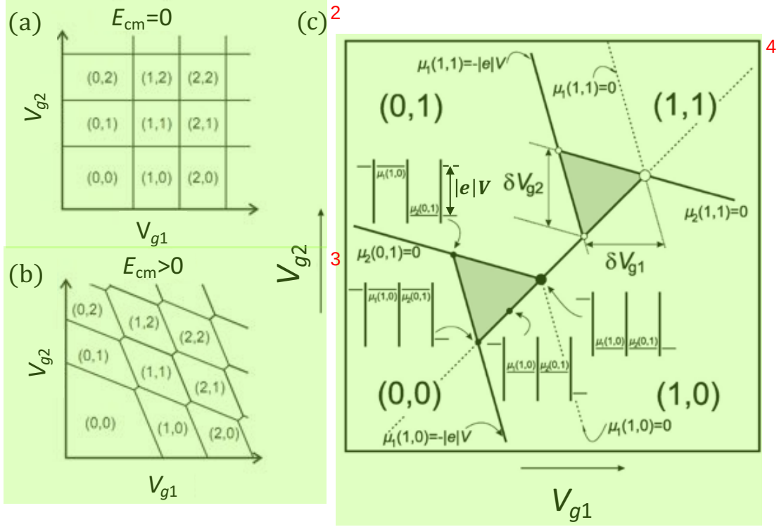
图 1.3 常相互作用模型下双量子点的电荷稳态图。(a) 无偏置电压时两个量子点之间不存在耦合的情况。(b) 无偏置电压时两个量子点之间耦合较大的情况。(c) 外加偏压时的电荷图，存在一对“偏压三角形”。图片来自 [28]。 5
