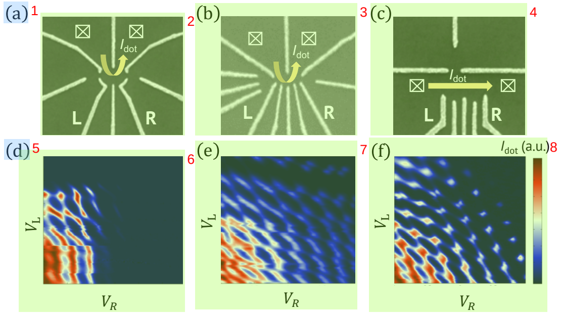
图 3.2 (a) ~ (c) 三种不同电极结构量子点的扫描电子显微镜图片。(d) ~ (f) 三种结构对应的电荷稳态图。结构中 I_{\text{dot}} 表示量子点中的电流导通沟道。白色带叉方块代表欧姆接触。
