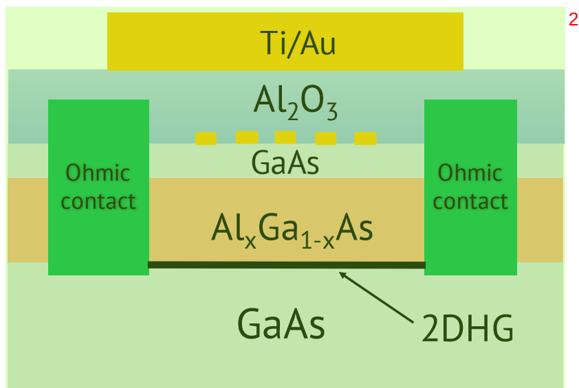
图 3.1 空穴型砷化镓的双量子点截面示意图 3
