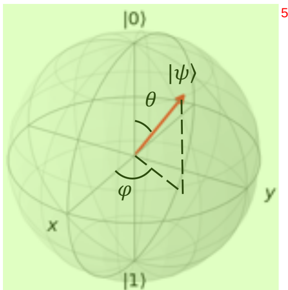
图 1.6 布洛赫球。北极为基态，南极为激发态。球面上任意一点对应的态矢为 |\psi\rangle = \cos \frac{\theta}{2} |0\rangle + e^{i\varphi} \sin \frac{\theta}{2} |1\rangle 。 5
