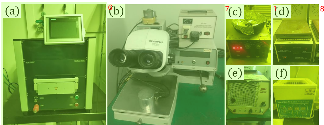
图 2.2 我们实验室使用的其他设备：(a) 退火炉。(b) 键合机。(c) 匀胶机。(d) 加热板。(e) 等 9 离子清洗机 (f) KQ-50DE 型超声仪。
